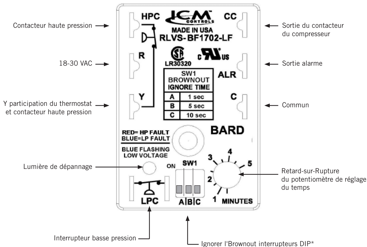
FIGURE 14 MODULE DE COMMANDE DU COMPRESSEUR
